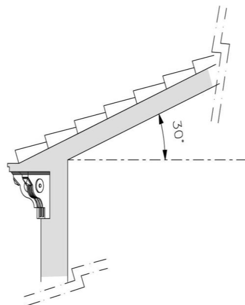
Toiture en tuile émaillée bleu Tamouda
