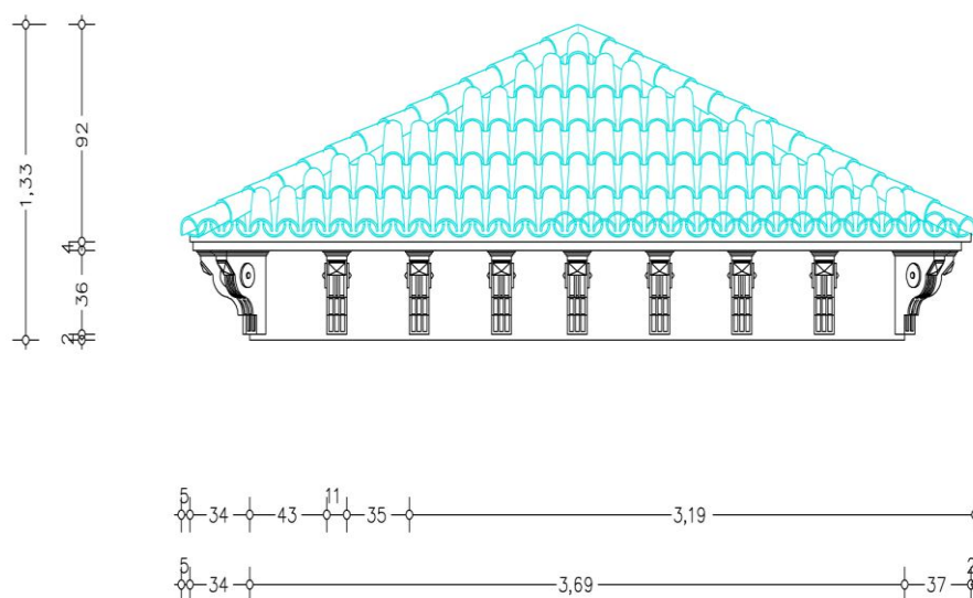
Détails de la Coupole de la Cage d'escalier
